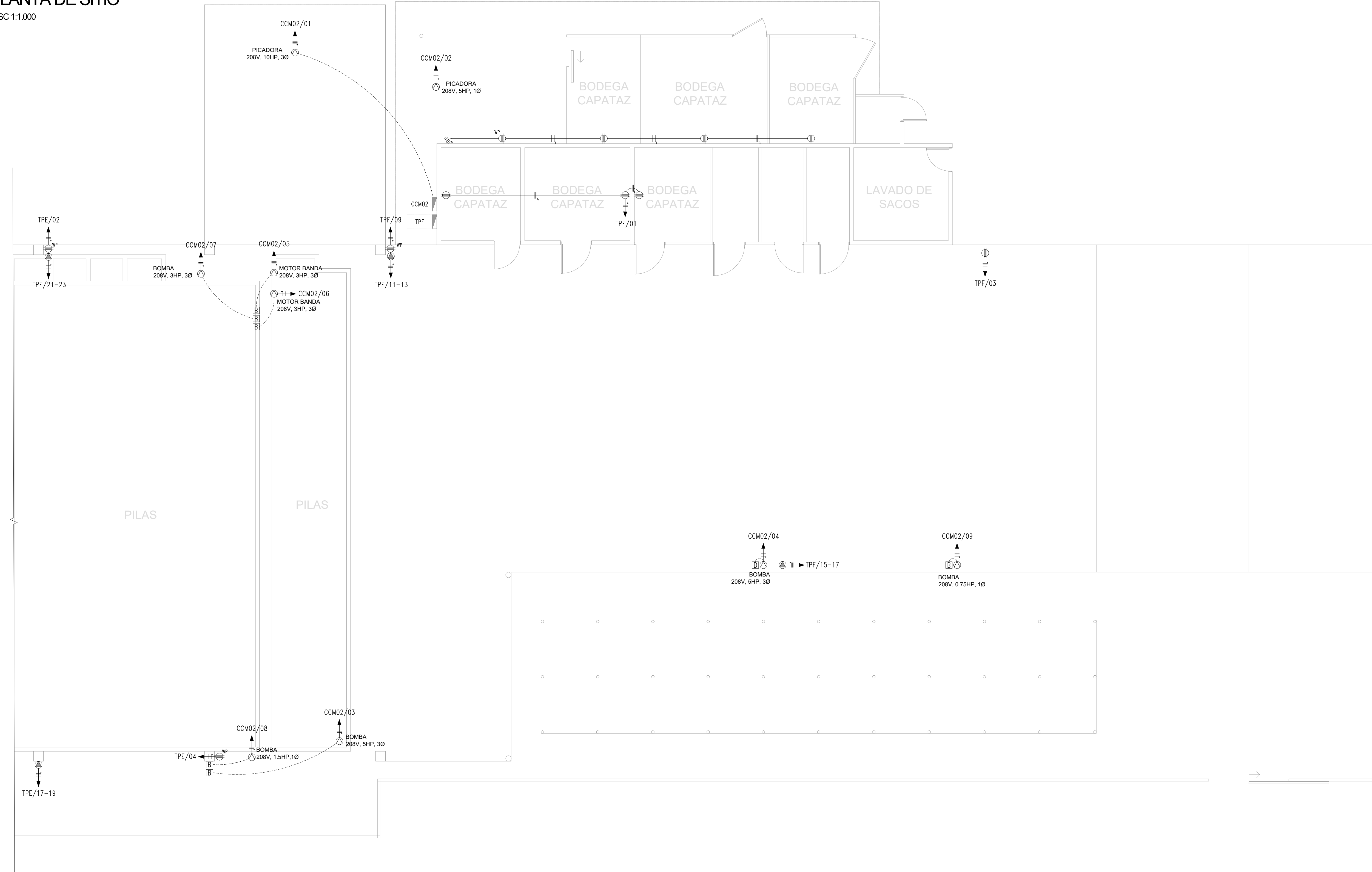
PLANTA DE DISTRIBUCIÓN DE TOMACORRIENTES Y EQUIPOS ELÉCTRICOS PLANTA DE EMPAQUE (SECCIÓN B) ESCALA 1:75
