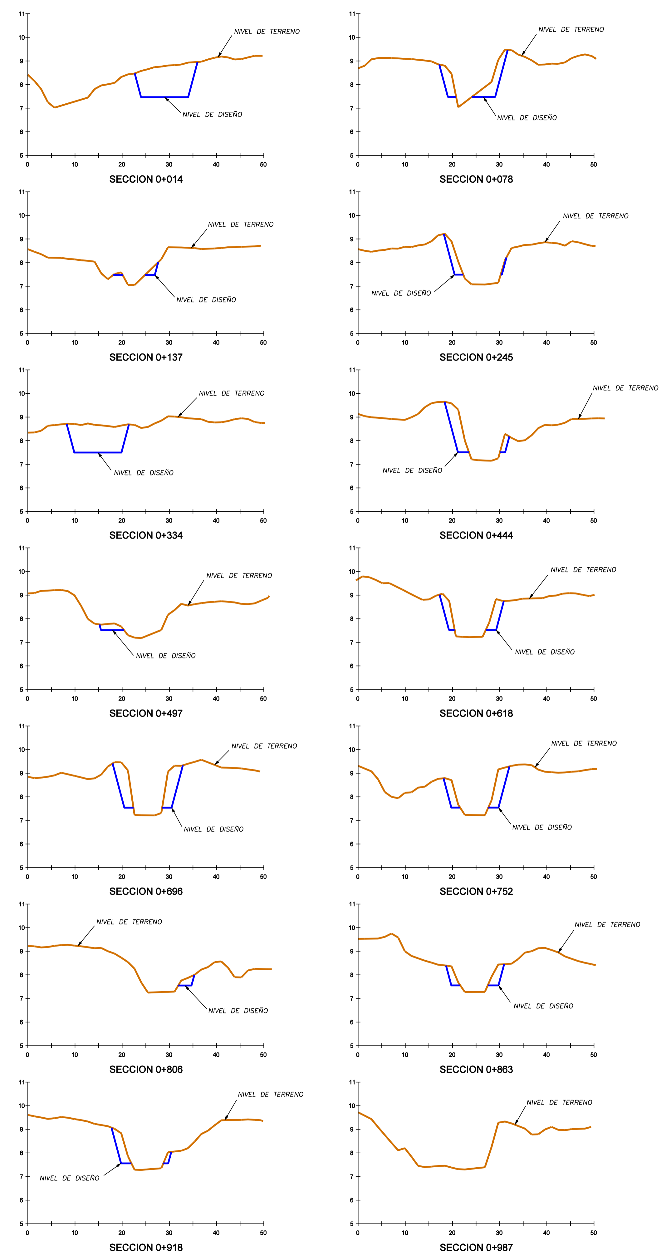
SECCIONES TRANSVERSALES ESCALA HORIZONTAL = 1:500 VERTICAL 1:100
