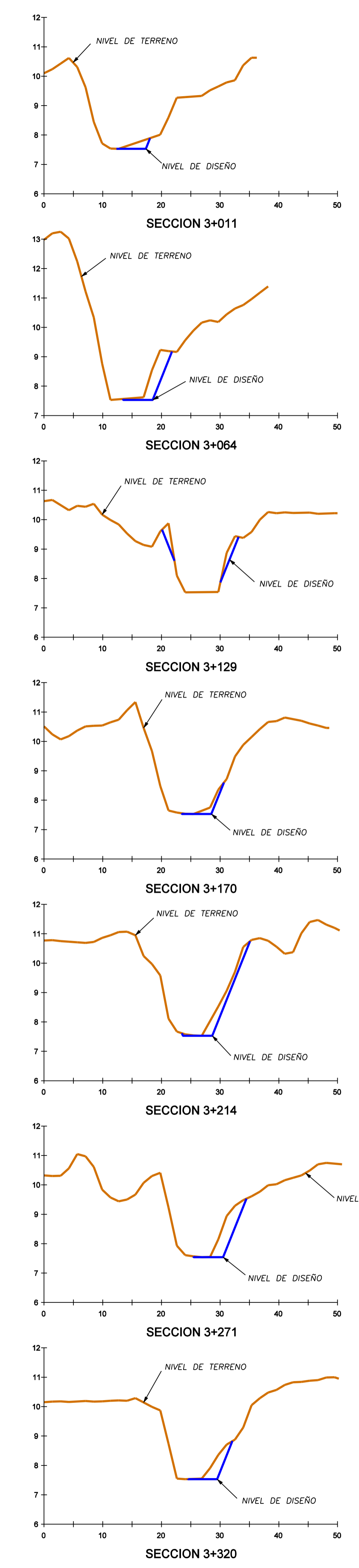
SECCIONES TRANSVERSALES ESCALA HORIZONTAL - 1:500 VERTICAL 1:100
