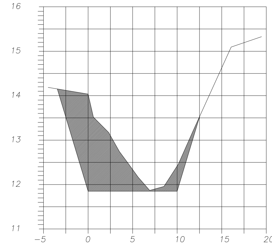
SECCION 47 EST 0+238 CANAL LLAMADA
