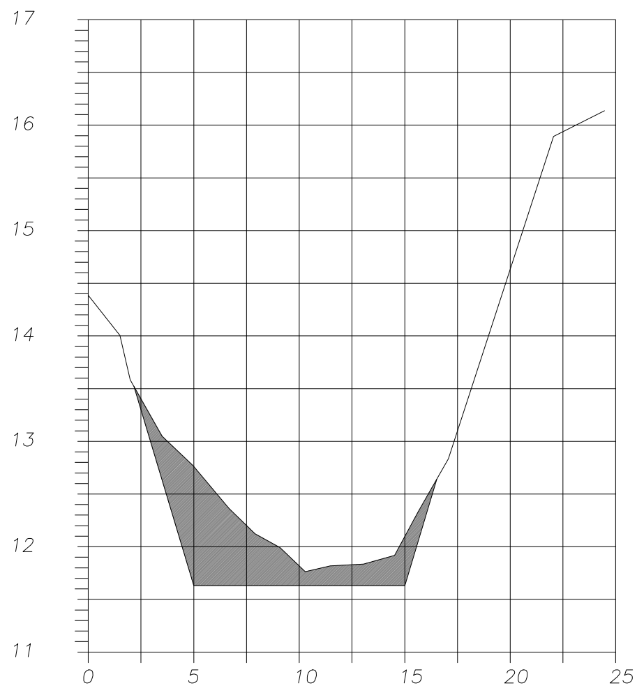
SECCION 58 EST 0+613 CANAL LLAMADA
