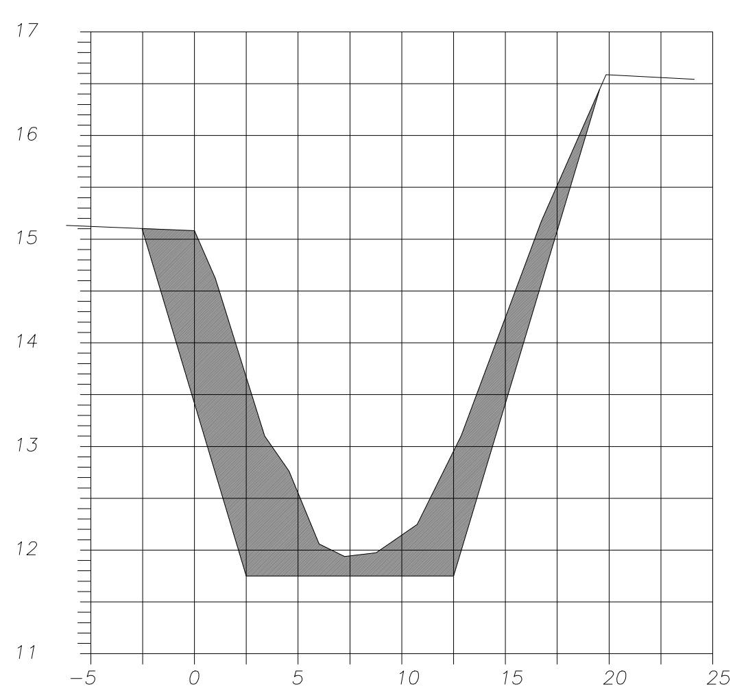
SECCION 52 EST 0+409 CANAL LLAMADA
