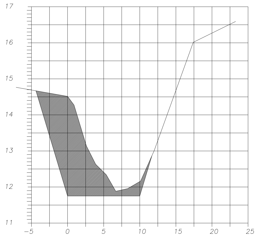
SECCION 51 EST 0+375 CANAL LLAMADA
