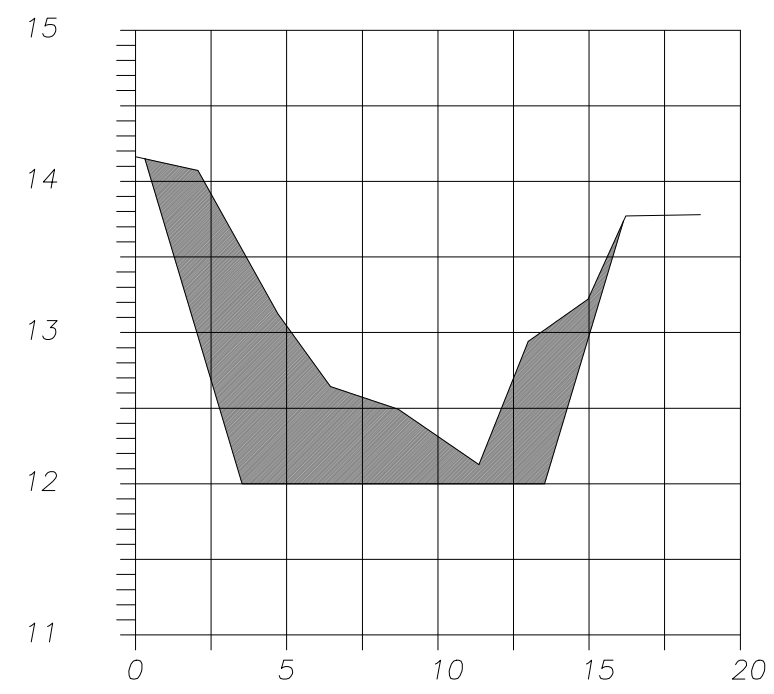
SECCION 40 EST 0+000 CANAL LLAMADA
