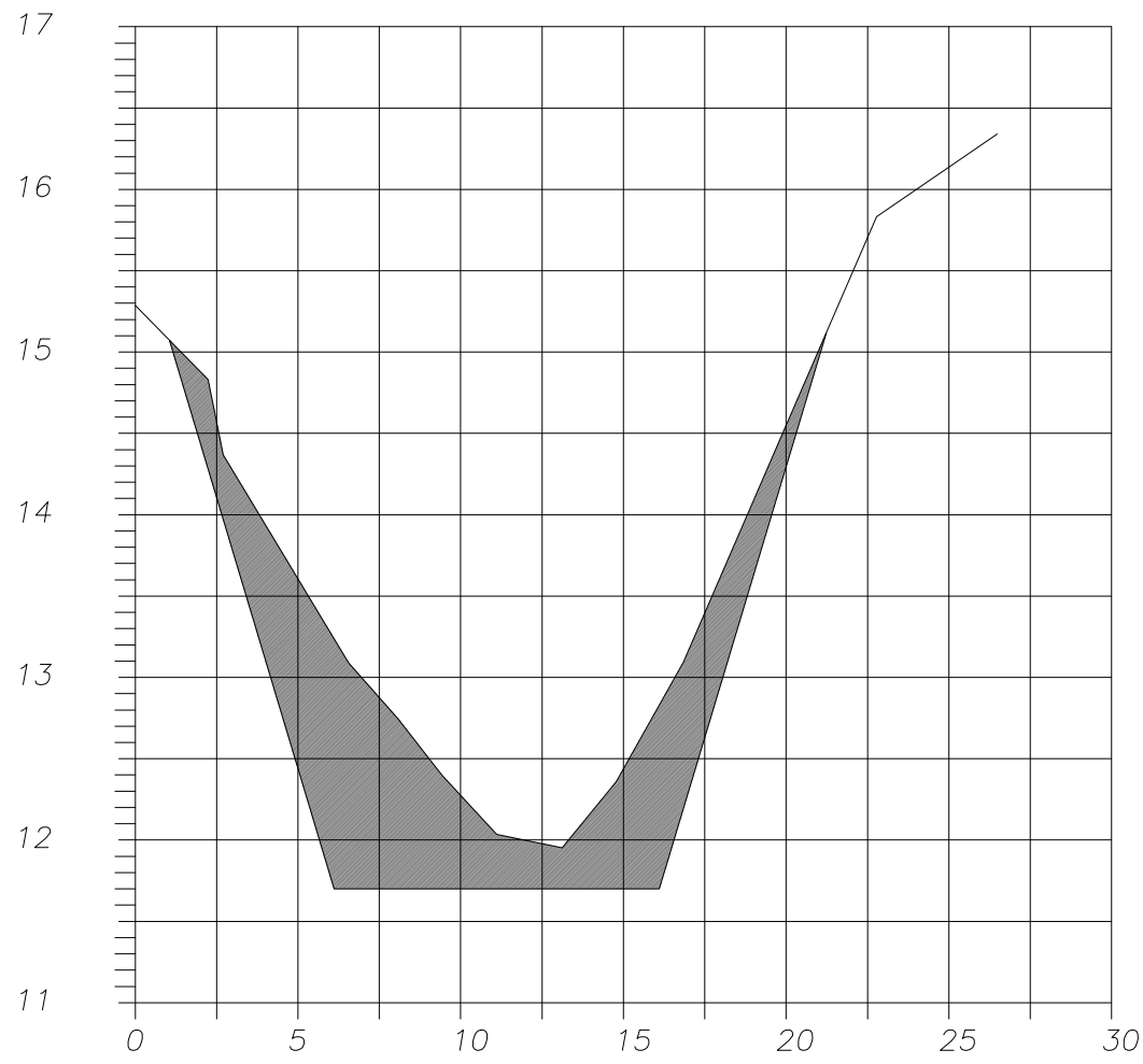
SECCION 55 EST 0+516 CANAL LLAMADA
