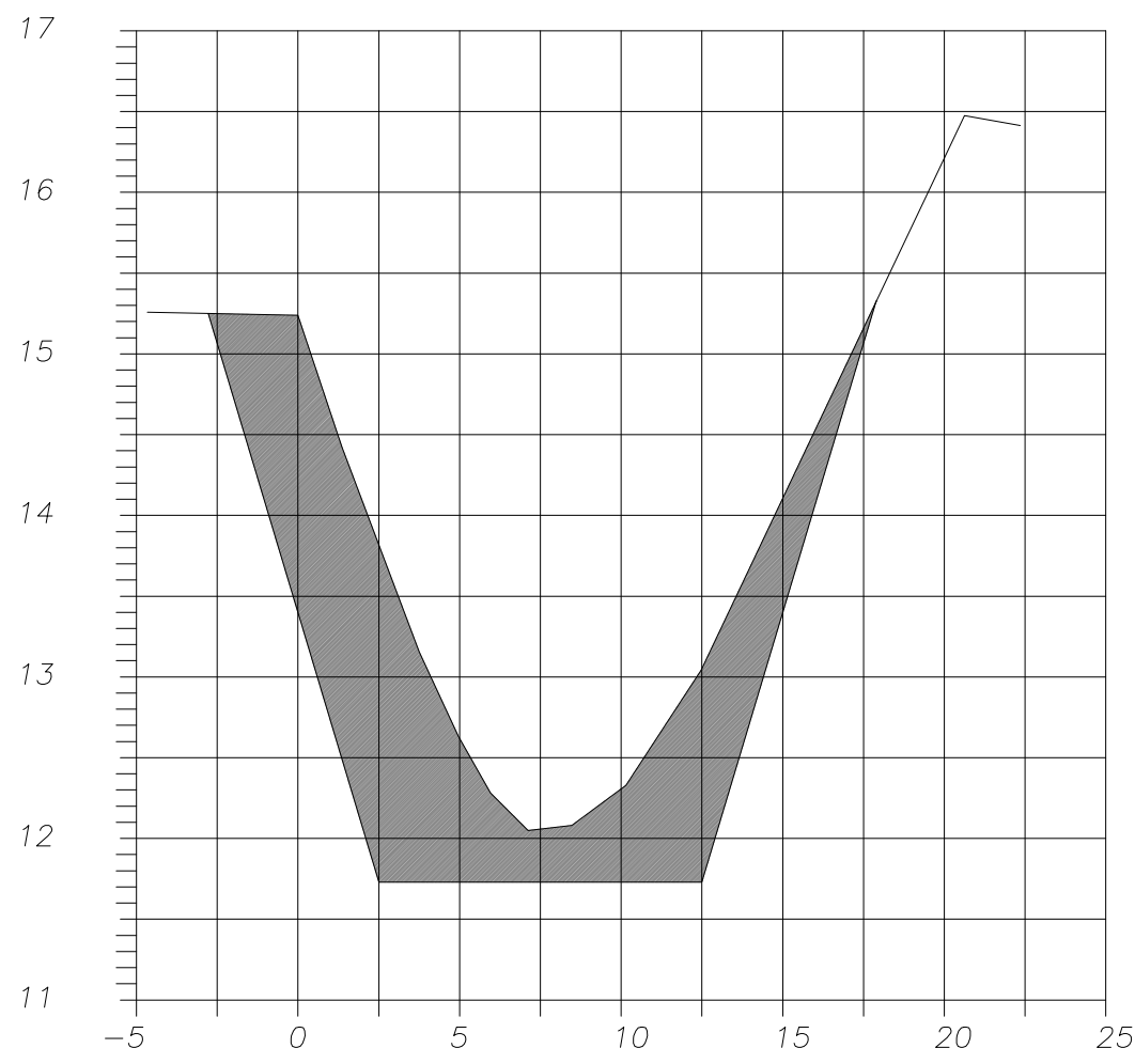
SECCION 53 EST 0+444 CANAL LLAMADA
