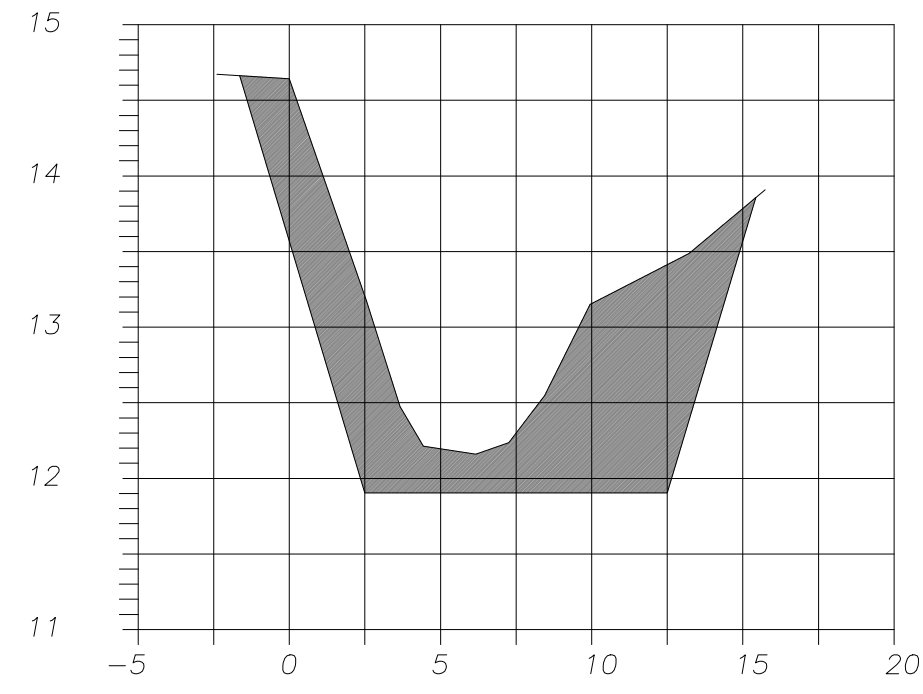
SECCION 43 EST 0+114 CANAL LLAMADA
