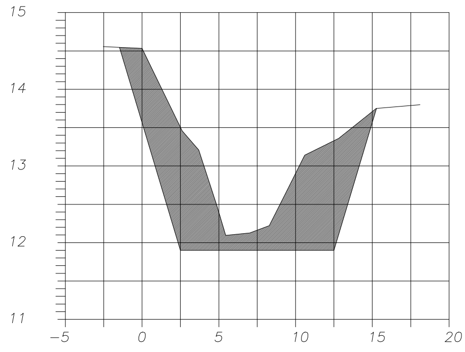
SECCION 44 EST 0+139 CANAL LLAMADA
