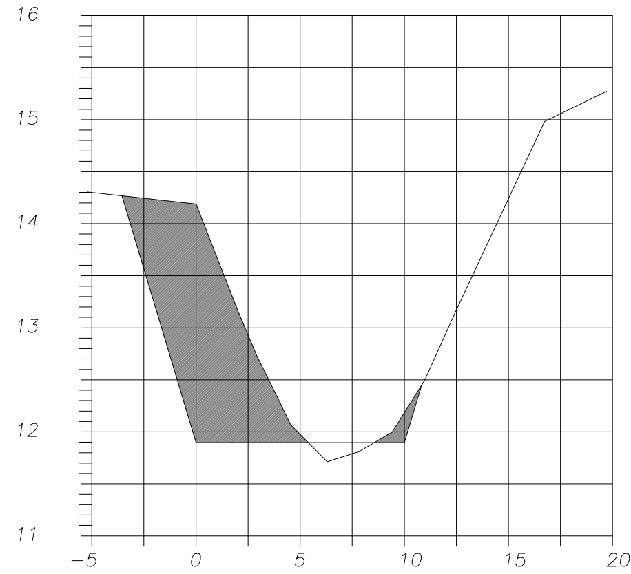
SECCION 46 EST 0+210 CANAL LLAMADA
