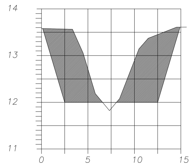
SECCION 41 EST 0+042 CANAL LLAMADA
