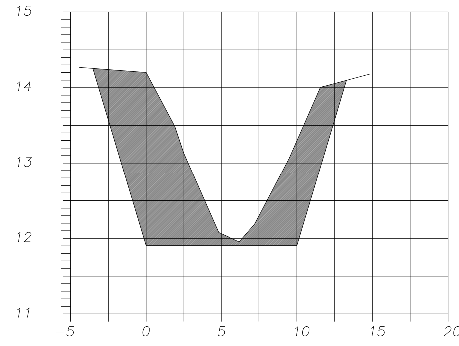
SECCION 45 EST 0+175 CANAL LLAMADA
