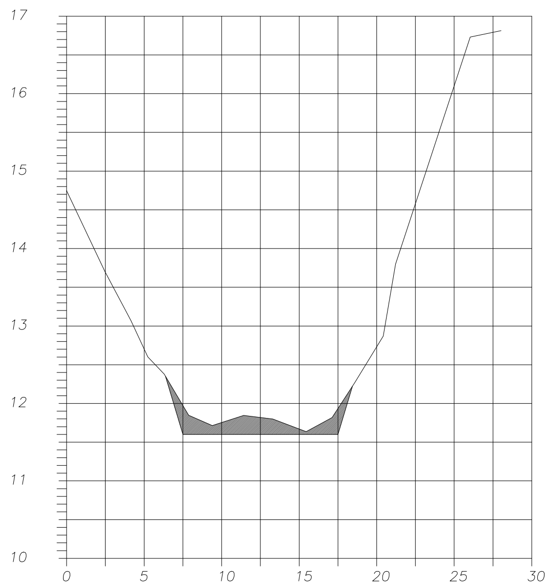
SECCION 59 EST 0+639 CANAL LLAMADA
