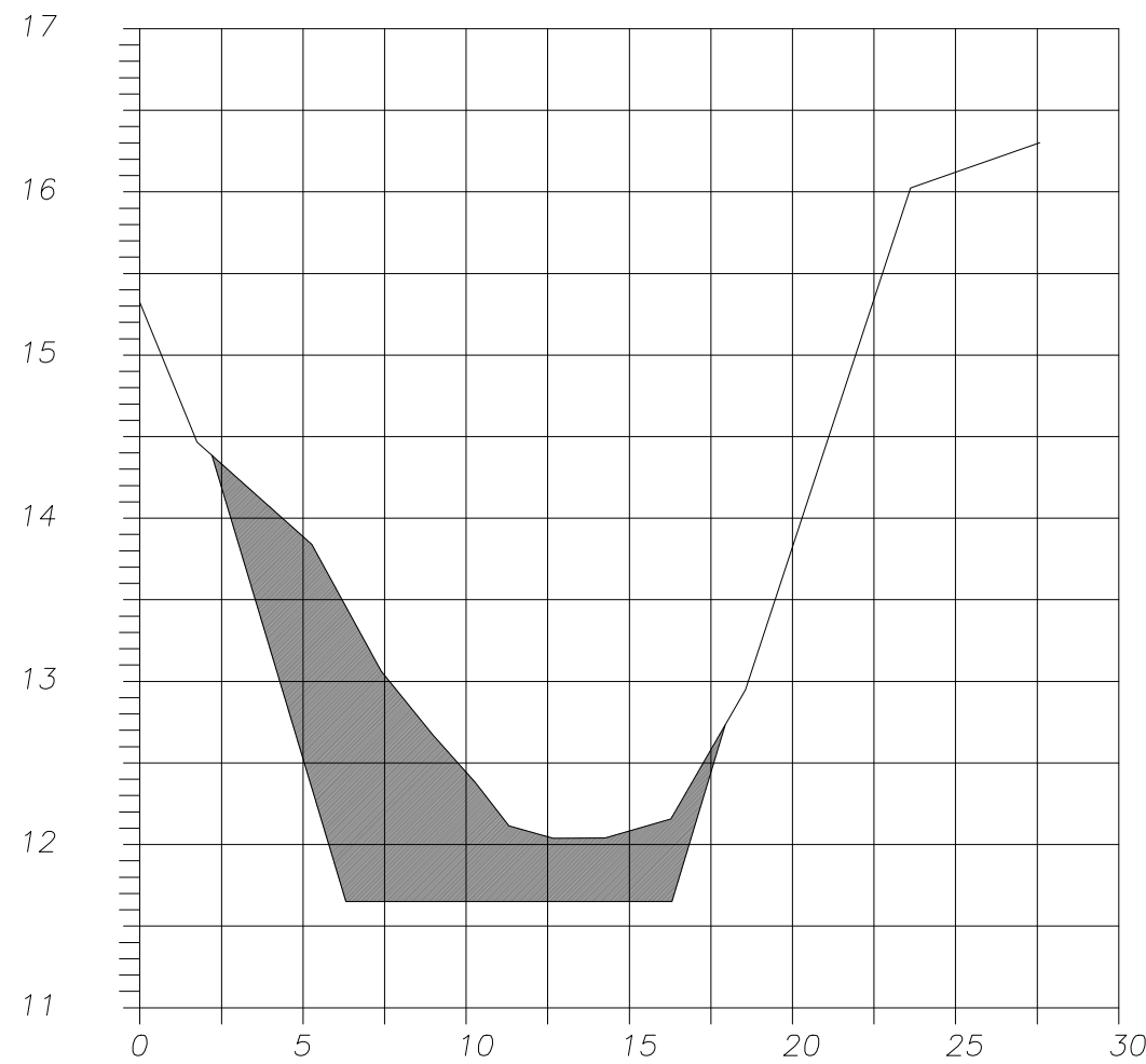
SECCION 57 EST 0+578 CANAL LLAMADA
