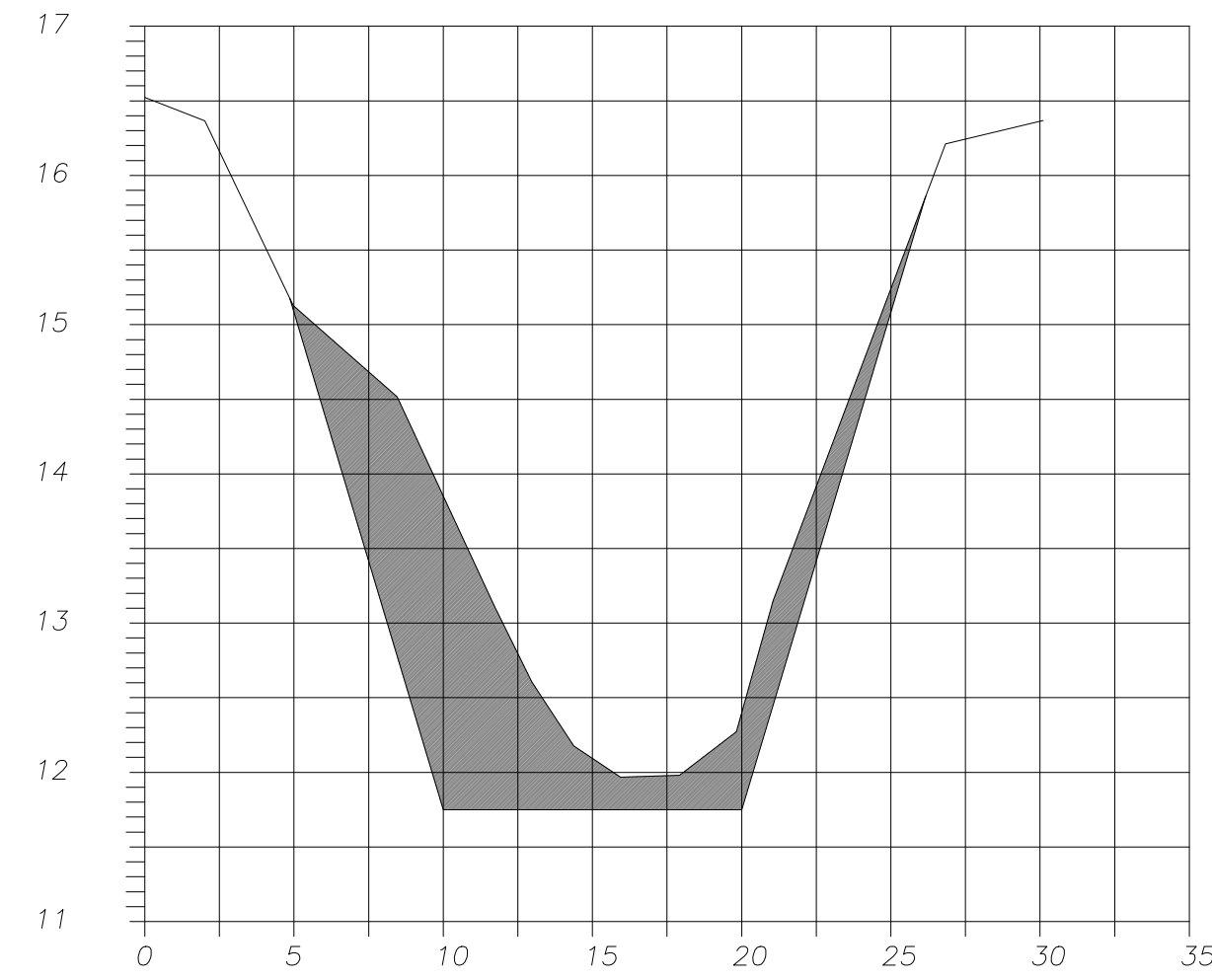
SECCION 50 EST 0+340 CANAL LLAMADA
