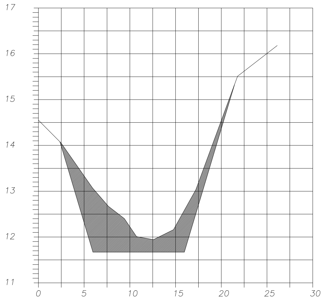
SECCION 56 EST 0+545 CANAL LLAMADA
