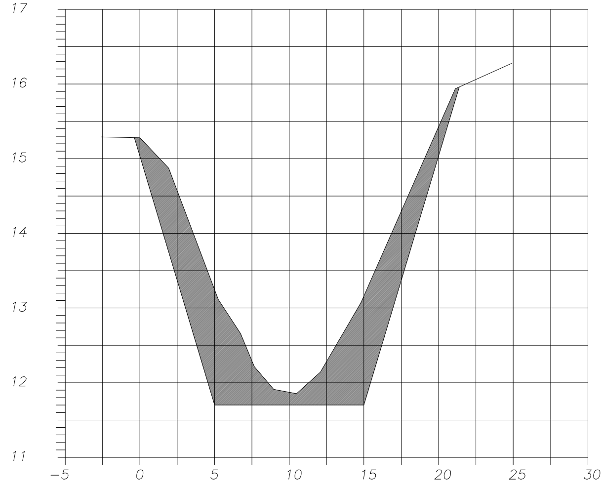
SECCION 54 EST 0+479 CANAL LLAMADA
