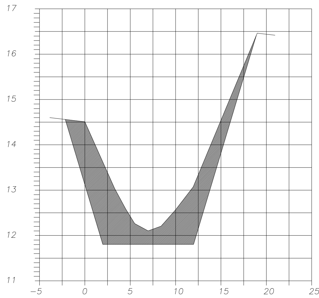
SECCION 49 EST 0+303 CANAL LLAMADA
