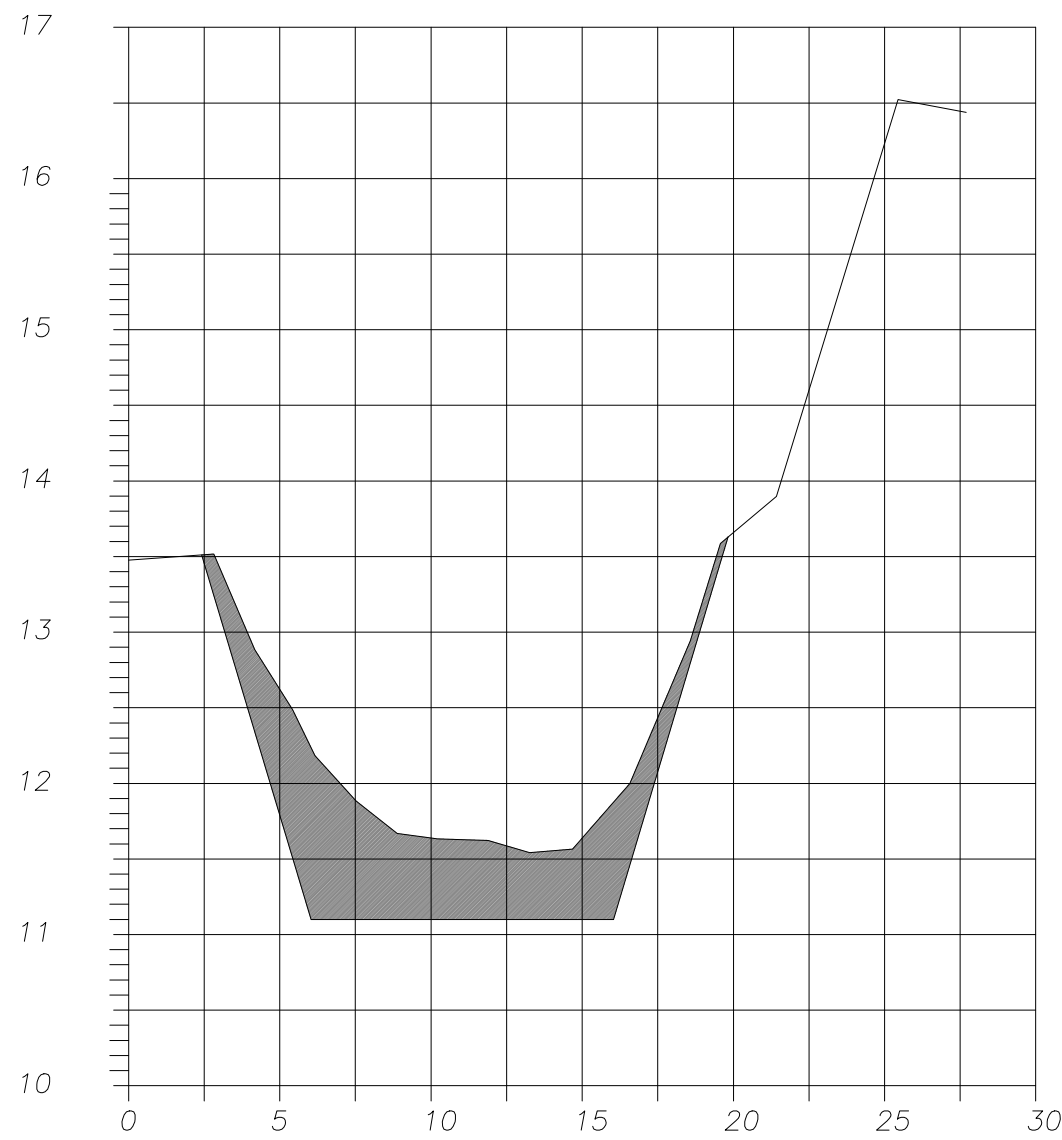
SECCION 60 EST 0+670 CANAL LLAMADA
