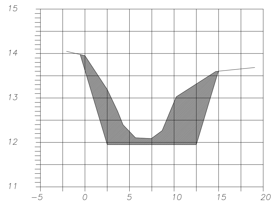
SECCION 42 EST 0+083 CANAL LLAMADA
