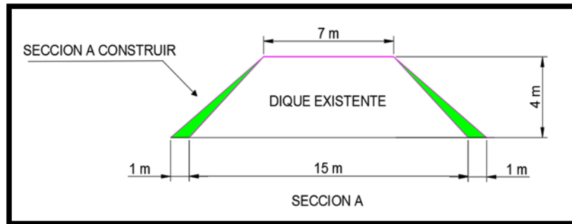
Figura 3. Sección transversal de los tramos de dique a reconformar en el dique de Matina.
