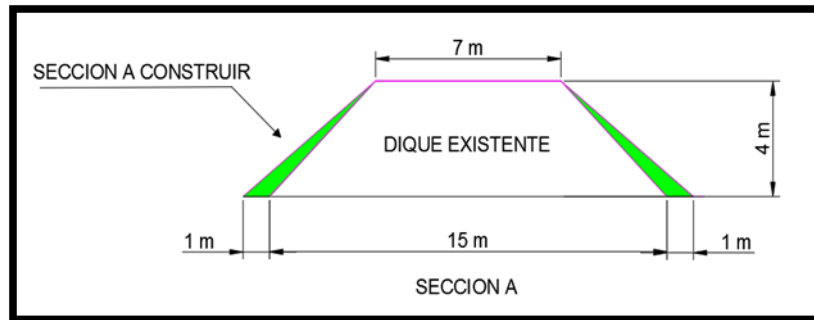
Figura 5. Sección transversal de los tramos de dique a reconformar en el dique de Estrada.
