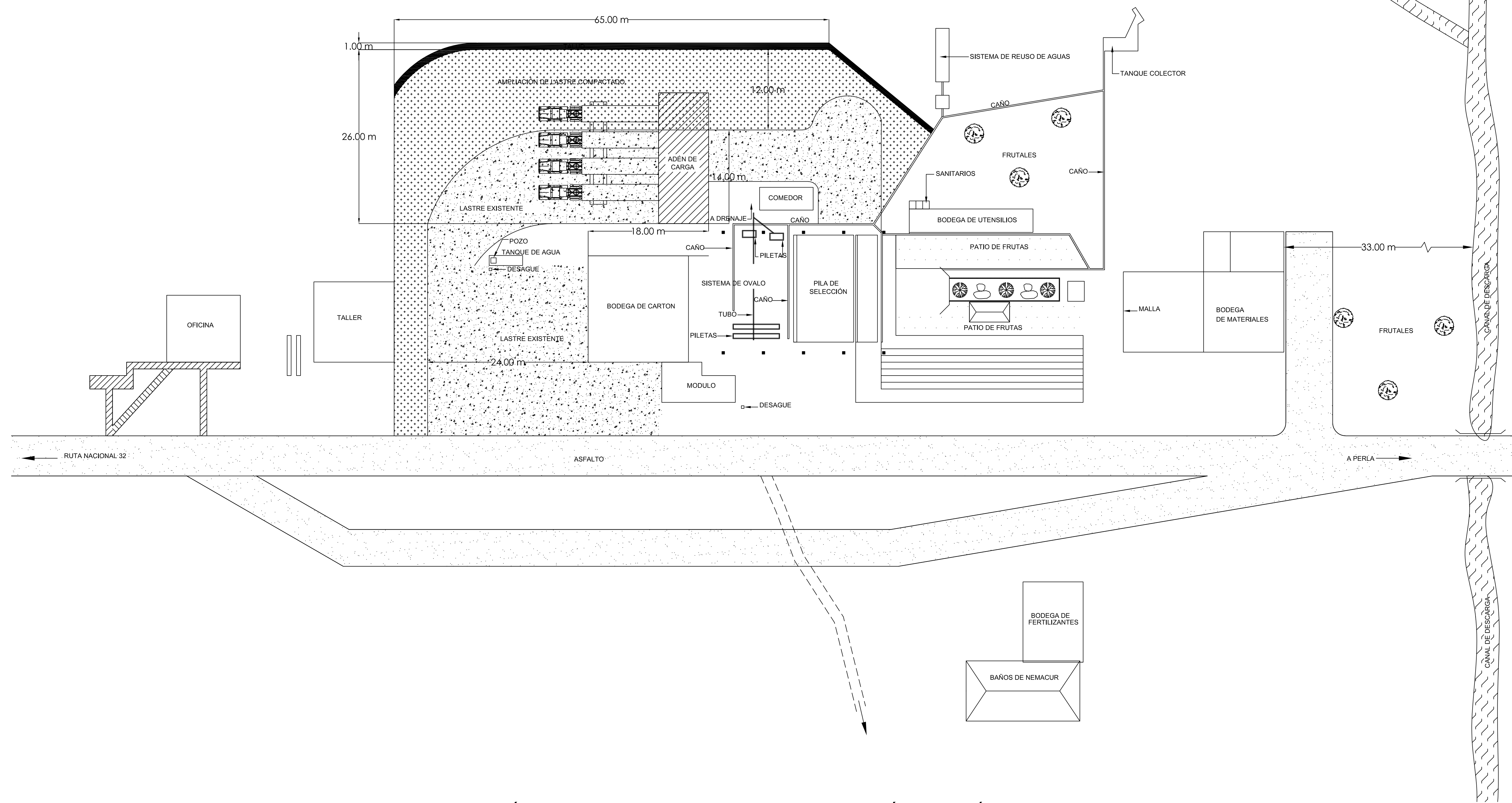
AMPLIACIÓN DEL CAMINO EN LASTRE COMPACTADO Y UBICACIÓN DEL ANDÉN DE CARGA ESCALA 1:300
