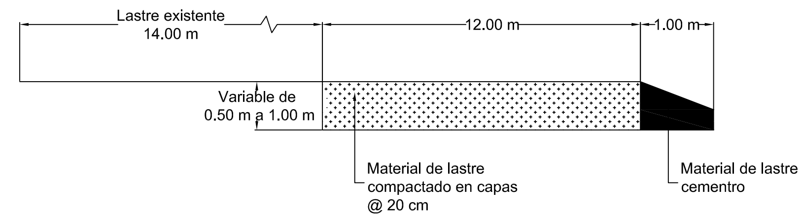
DETALLE DE AMPLIACIÓN DEL CAMINO EN LASTRE COMPACTADO ESCALA 1:50
