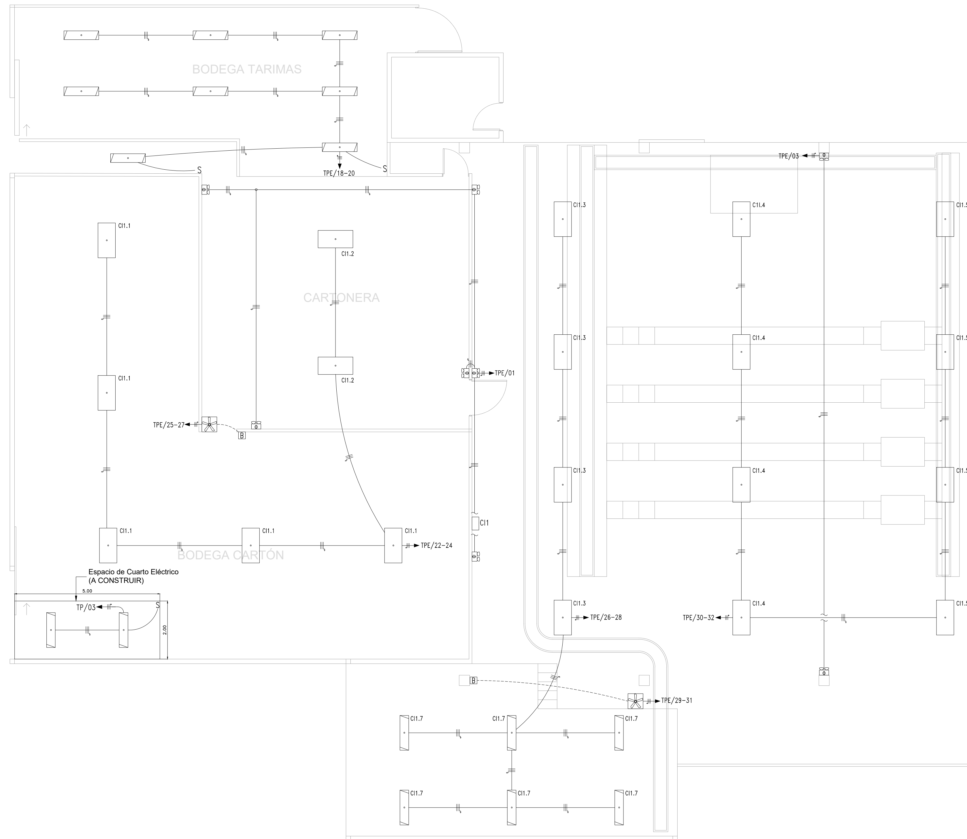
PLANTA DE DISTRIBUCIÓN DE LUMINARIAS PLANTA DE EMPAQUE (SECCIÓN A) ESCALA 1:75
